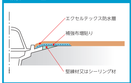
■横引きドレン回り
