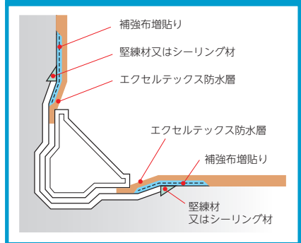
■横引きドレン回り
